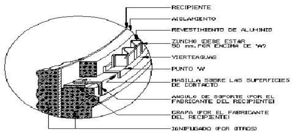
DETALLE "B"
