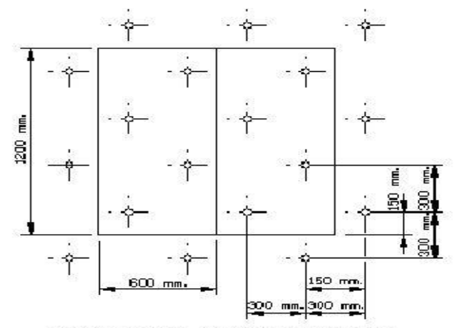
DISPOSICION DE LOS PASADORES PARA SOPORTAR MANTAS DE 600 mm. x 3200 mm. LOS PASADORES NO TENDRAN MENOS DE 10 6A DE DIAMETRO.
