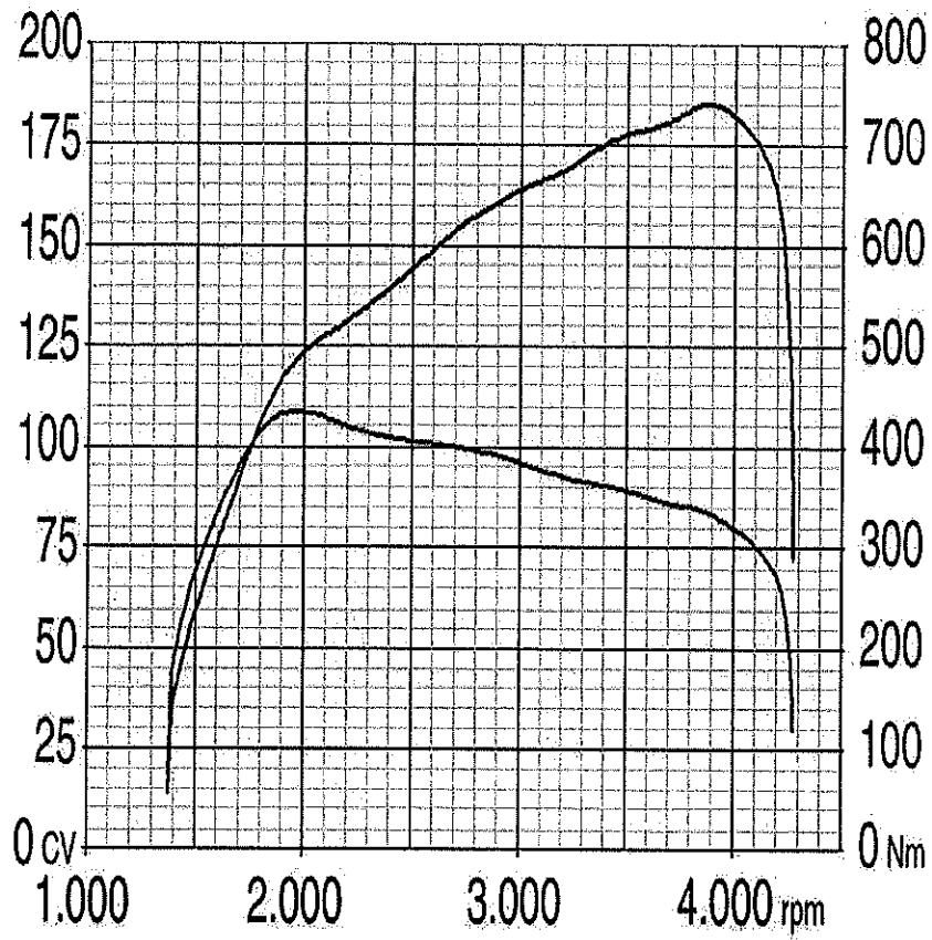
CURVA DE POTENCIA AMAROK HIGHLINE 4X2 MANUAL, 4X4 MANUAL 2.0 180CV
