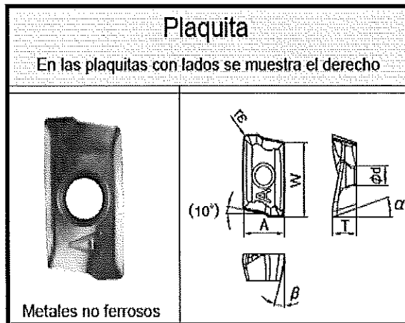
Figura 1. Plaqueta de fresado
